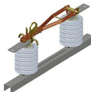
Chave Seccionadora Unipolar Polimérica
